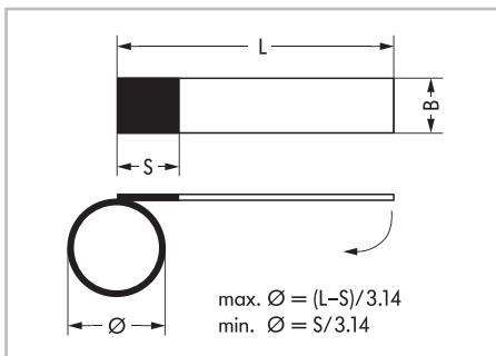
不干胶标签的外形尺寸(单位：mm)
