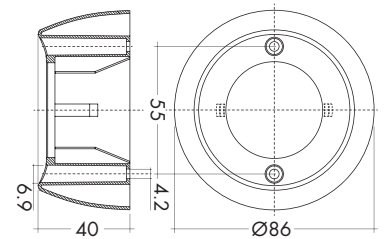
外置安装
