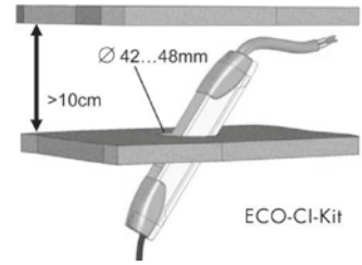
ECO CI组件
