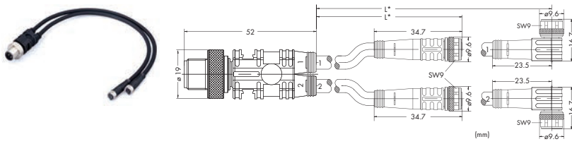
M12分支电缆针式接头
