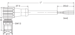
M12针式接头
