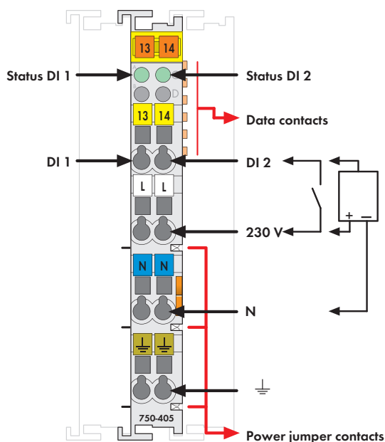
图: 750系列 该型号不包含小型WSB标记系列 该数字量输入模块可接收现场侧(如: 传感器等)的控制信号。
