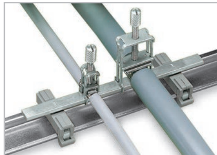
汇流条，带有2个接地脚 长度125 mm，汇流条与导轨平行 型号：790-115
