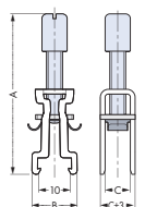
初始状态可直接安装
