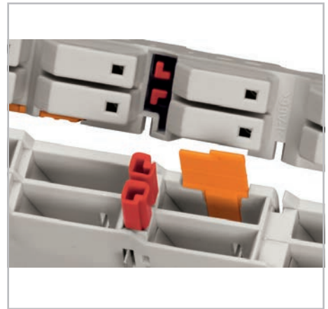
通过定位销挡块实现对可插拔前连接器的防插错保护(选配)
