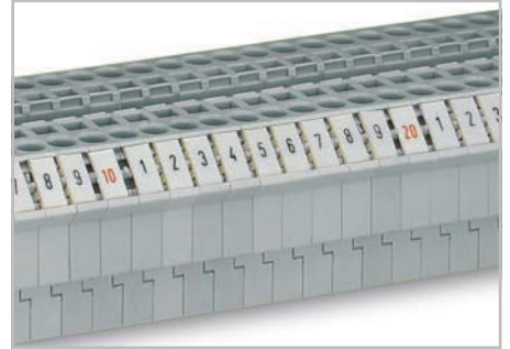
使用WMB十个一组的标记牌
