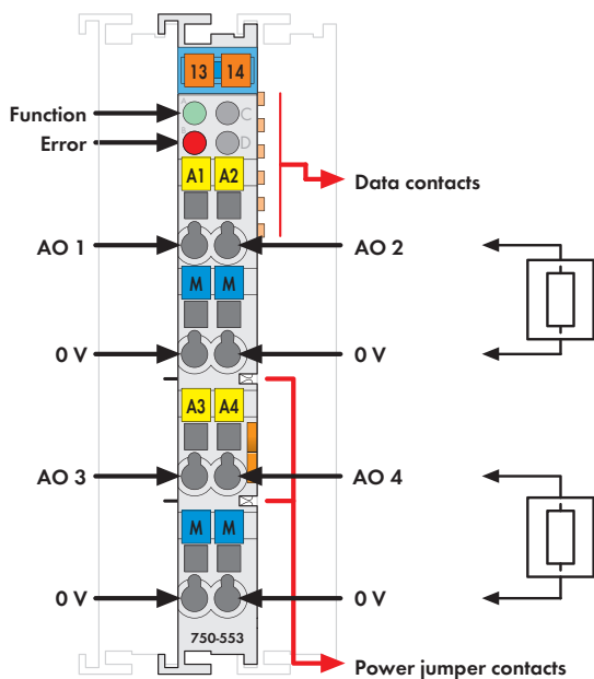
图: 750系列 该型号不包含小型WSB标记系列 该模拟量输出模块可输出产生0-20mA或4-20mA标准信号。 输出信号经电气隔离,并以12位分辨率的形式传输。 电流型模拟量输出模块由现场侧电源供电(环路供电)。
