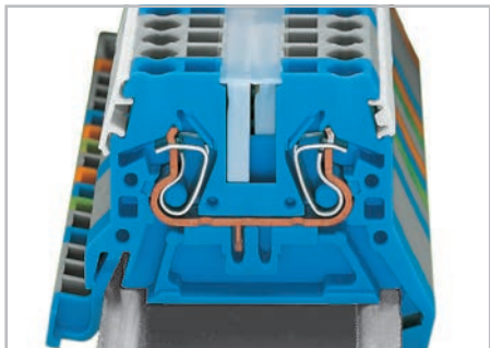
小型WSB标记牌 在小型WSB标记位安装WMB标记牌 标记条，半透明
